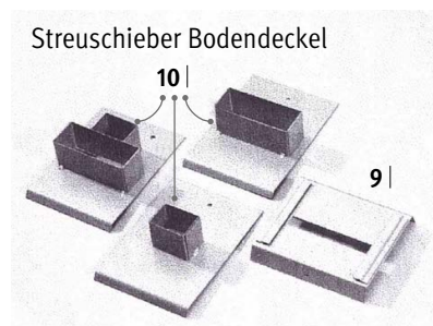
Zu 10: Ausführungen der Streuschieber Modelle: 502/506/505
